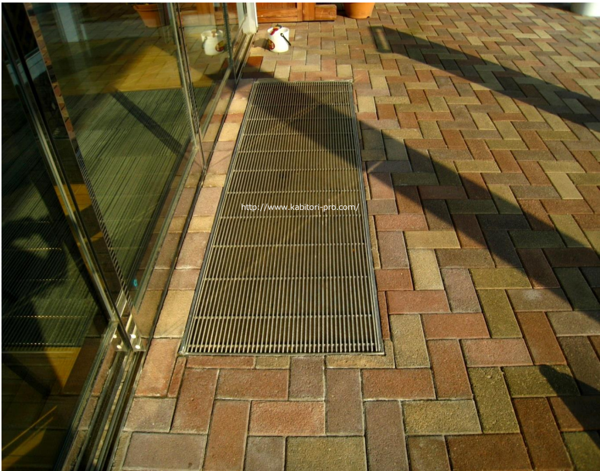
施工後
